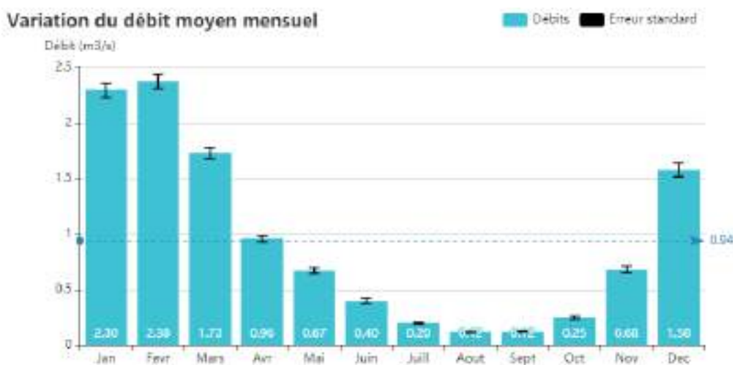
Figure 72 : Variation du débit moyen mensuel (station M6323010)
