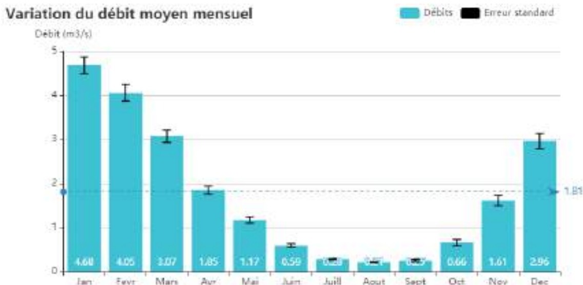
Figure 75 : Variation du débit moyen mensuel (station M6333030)
